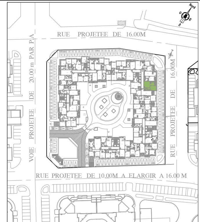
PLAN 4ème ETAGE
