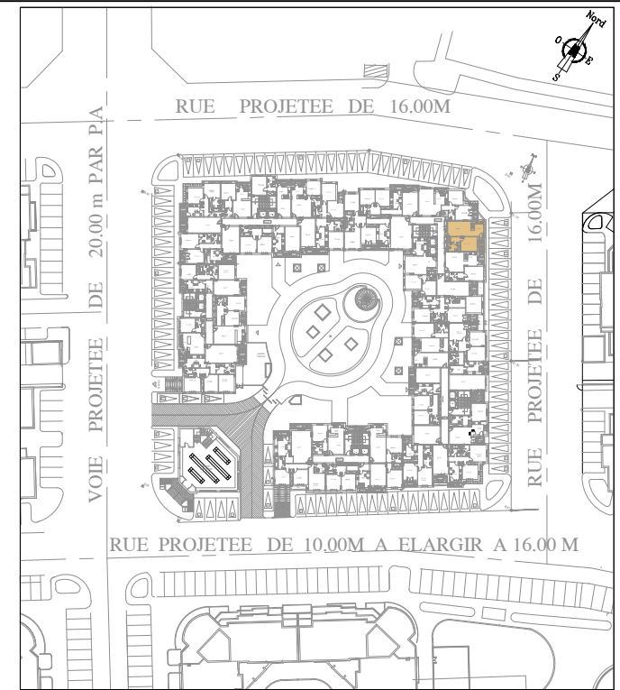
PLAN 1 er ETAGE
