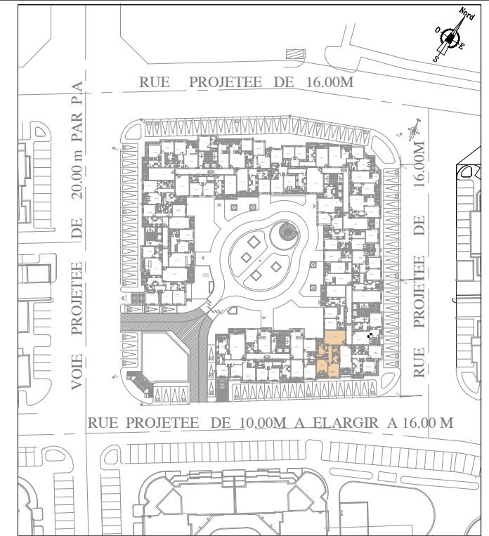
PLAN 2ème ETAGE
