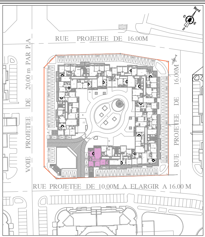
PLAN 6ème ETAGE
