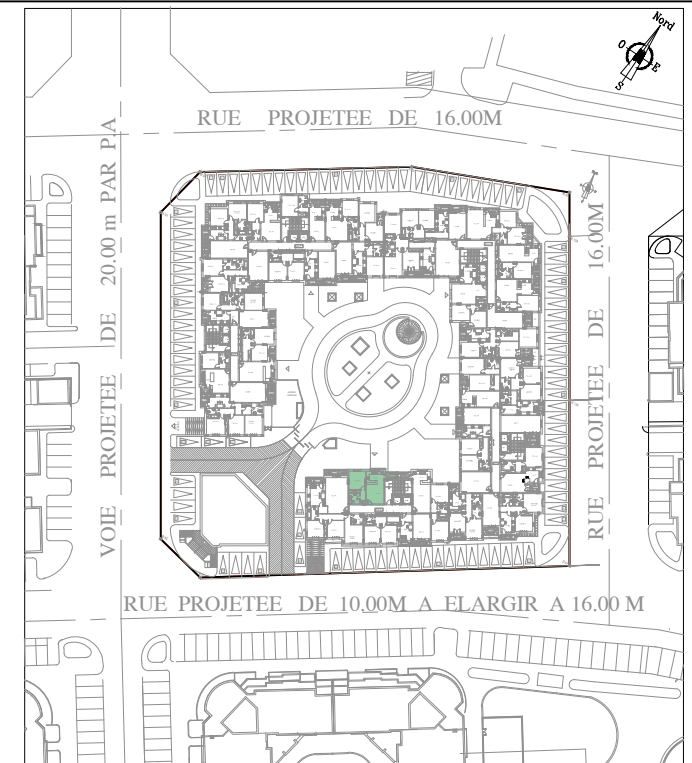
PLAN 5ème ETAGE
